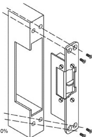
木門安裝圖
