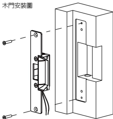
木門安裝圖
