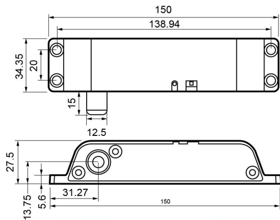
上方安裝
