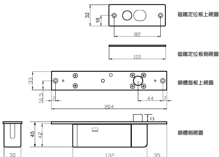
尺寸圖 單位:公厘
