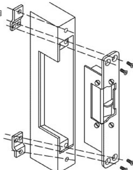
金屬門安裝圖
