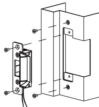
金屬門安裝圖
